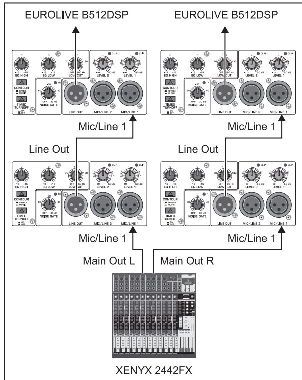
Fig. 3.3: Conexión en serie de varios B512DSP
